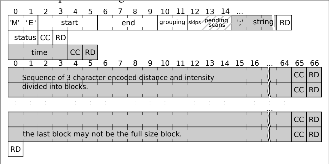
Figure 3.7 : ME Message Format
