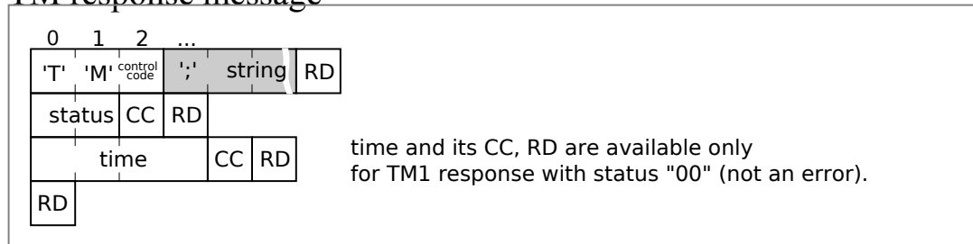
Figure 3.17 : TM Message Format
