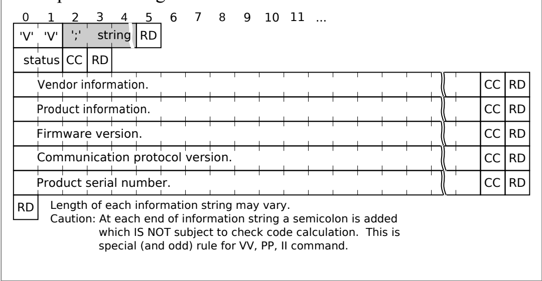
Figure 3.18 : VV Message Format
