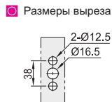
Размеры выреза
