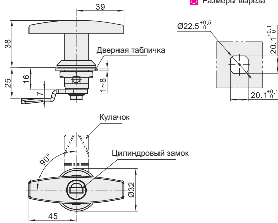
Размеры выреза
