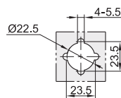
Размеры выреза
