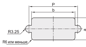
Размеры выреза
