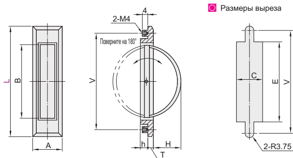
Размеры выреза
