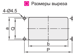
Размеры выреза
