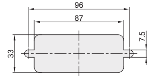
Размеры выреза
