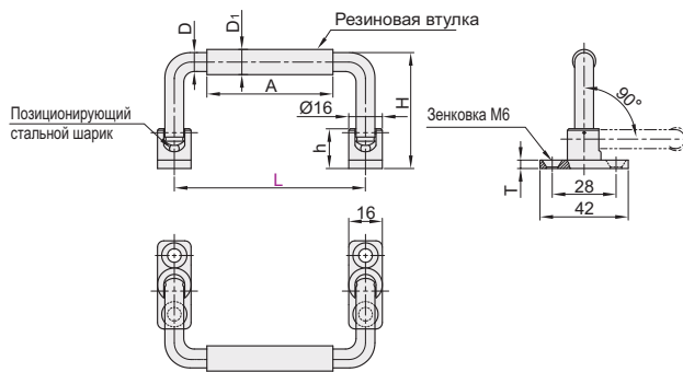
Раззенкованное отверстие XAN01
