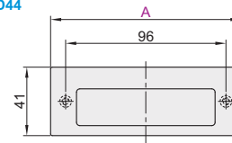
Размеры выреза
