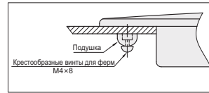
Монтажный чертеж
