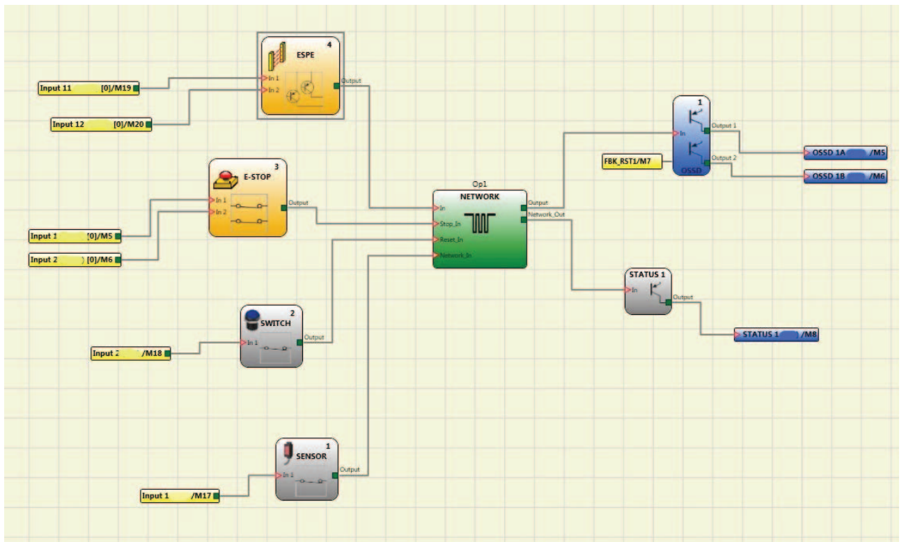
Figure 48 – Exemple d'utilisation du bloc NETWORK
