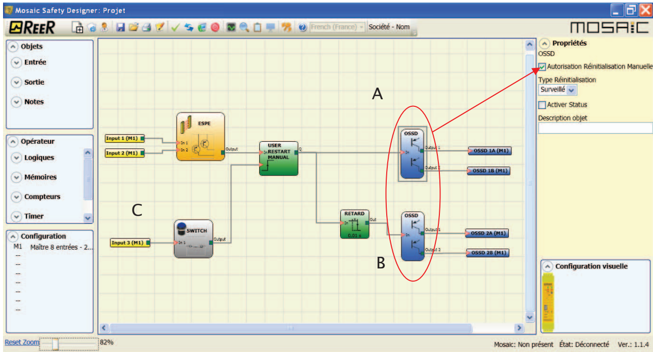
Figure 49 – Double sortie avec la seconde retardée en Manuel
