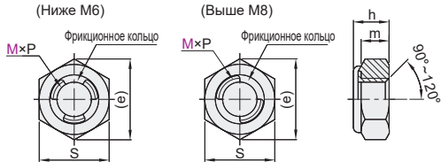
U-образная гайка (металлическое фрикционное кольцо) ТВК42
