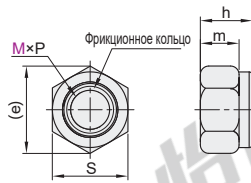
U-образная гайка (пластиковое фрикционное кольцо) ТВК44
