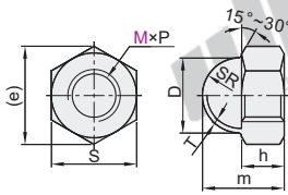
Куполообразная гайка ТВК11
