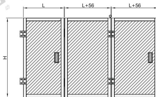
Размер открывания дверной коробки
