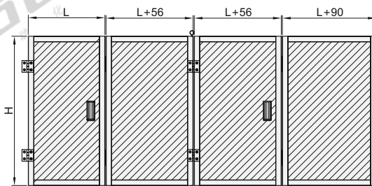
Размер открывания дверной коробки
