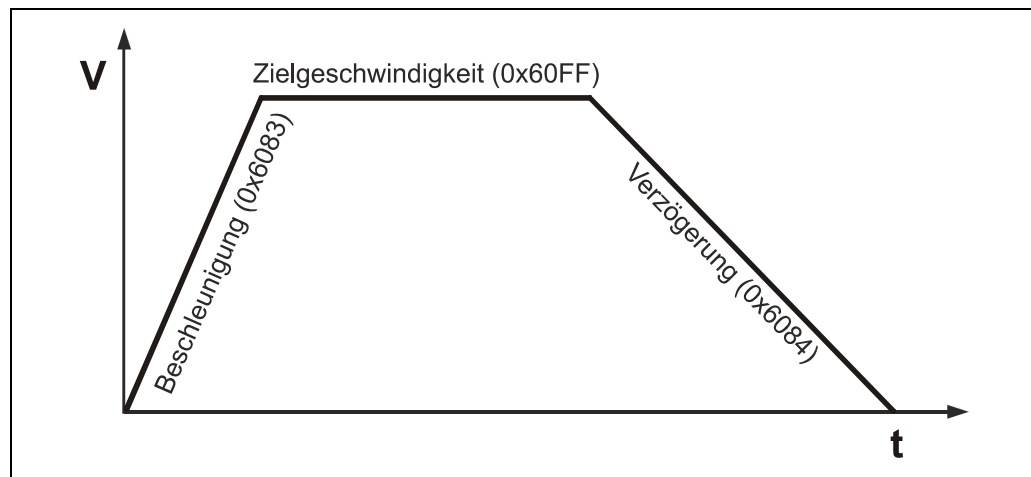
Abbildung 11: Geschwindigkeitsrampe
